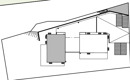
Villa 1 Rez-de-chaussée - variante 1
